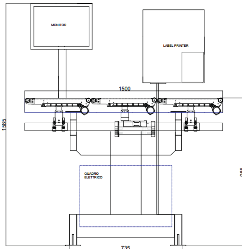
APPLICATORE DI ETICHETTA AIR BLAST / AIR BLAST LABEL APPLICATOR
